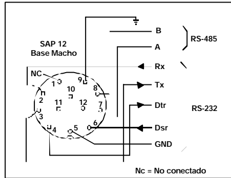
Conector SERIE para visualizadores DT-106X y DT-111X.
