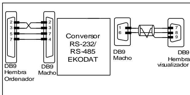
3.2.4a. Cable de conexión RS-485 entre los visualizadores DT-105X, DT-106X, DT-110X, DT-111X y DT-203X, un ordenador PC y un convertor CV-485 Ekodat.
