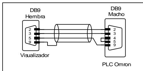
CONEXION ENTRE UN PLC OMRON Y UN DT-105X, DT-110X, DT-106, DT-111 o DT-203X
